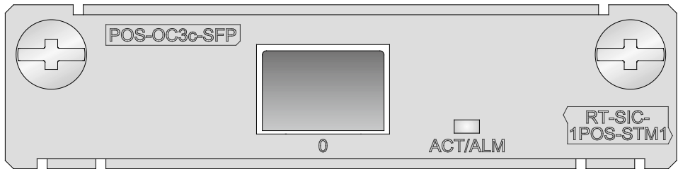
图1-2 RT-SIC-1POS-STM1 模块前面板
