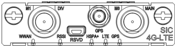
图1-6 SIC-4G-LTE-M 模块面板
